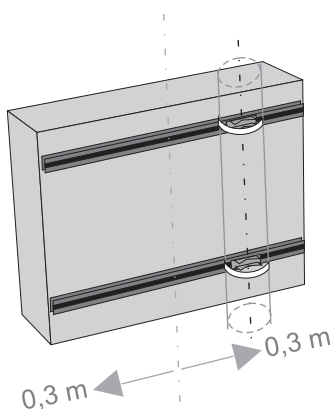
UCHYCENÍ POMOCÍ LIŠT S MOŽNOSTÍ VYVOSENÍ
